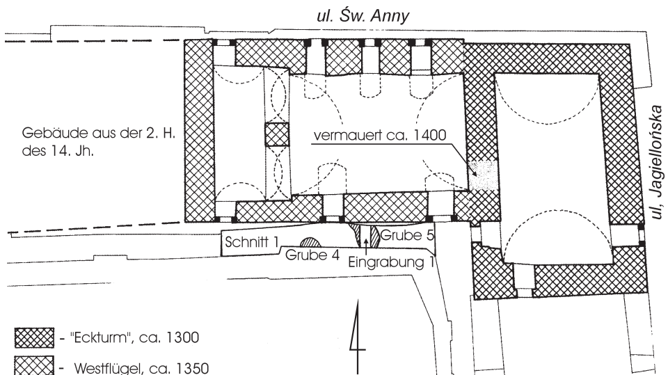
Abb. 1. Kraków, Stare Miasto, ul. Jagiellońska 15 - ul. Św. Anny 8. Planum der Kellerräume des Collegium Maius im Bereich des Peçherz-Hauses. Lage der Grabungsschnitte und Befunde. Zeichnung nach S. Sławiński, J. Hiżycka (2004, Abb. II.2) mit Ergänzungen von D. Niemiec.
